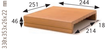
PASAMANOS INT. 21,5 HANDRAIL INT. 21,5
