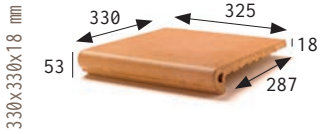
PELDAÑO REDONDEADO 33 ROUNDED STAIR-TREAD 33
