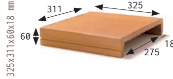
PASAMANOS INT. 27,5 HANDRAIL INT. 27,5
