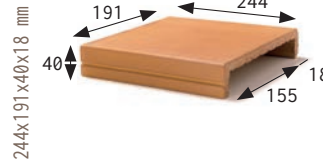
PASAMANOS INT. 15,5 HANDRAIL INT. 15,5
