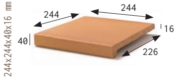
VIERTEAGUAS 25X25 NATURAL WASH 25X25
