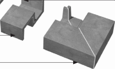
PIEZA MACIZA ESQUINA DE NICHOS/ANCLAJE CORCHERA NICHE CORNER PIECE/LANE ROPE FIXING PIECE
