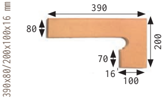
ZANQUÍN REDONDEADO DCHA. ROUNDED STRING RIGHT SIDE
