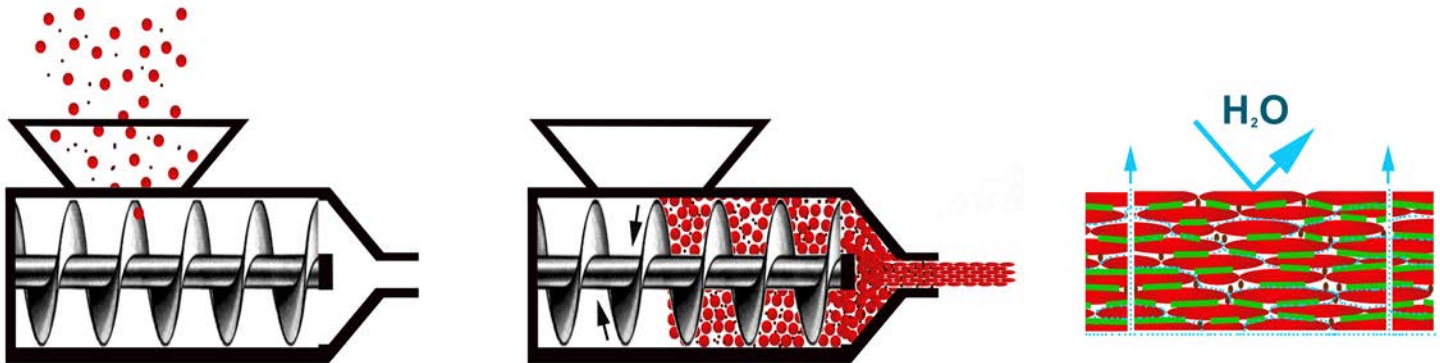
Proceso y estructura materiales extrudidos Gres Aragón. Process and structure of Gres Aragón extruded materials.
